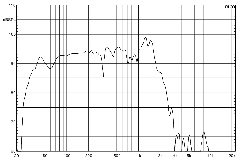
頻響曲綫
